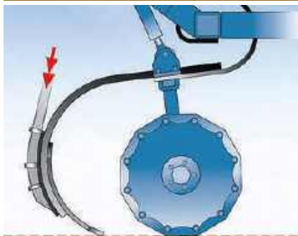
Рисунок 2: глубокая регулировка (цилиндр разжатый)
